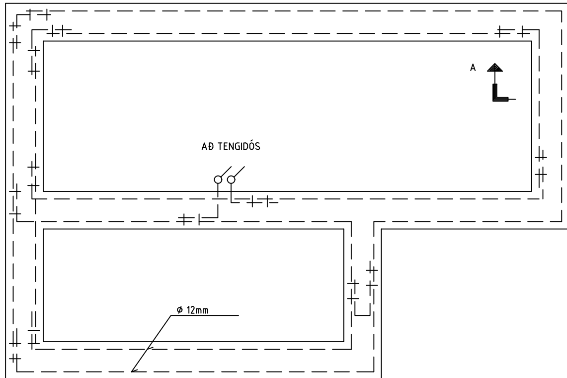
GRUNNMYND SÖKKULVEGGJA
